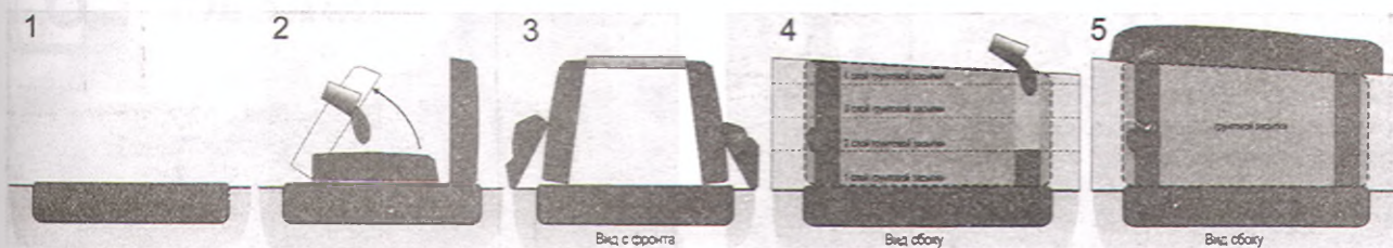
Рис. 9. Схема строительства кирпичного дольмена.
