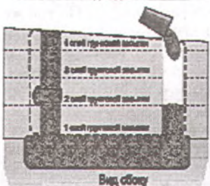
Р и с. 6. Формирование опалубки грунтовой засыпкой и заливка фронтальной и задней плит.
