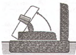
Р и с. 4. Заливка второй боковой плиты.
