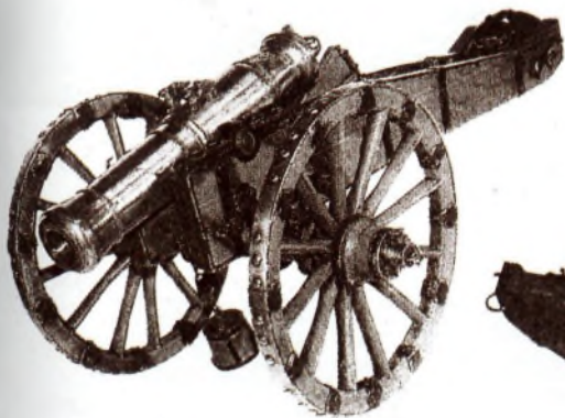
Секретная гаубица образца 1758 года (система П. И. Шувалова). По ней есть указание Сената: «Хранить в арсенале за печатью, дабы имеющаяся в ней инвенция (т.е. изобретение), кроме наружности НИКОМУ открыта быть не могла ».
