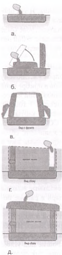
Рис. 1. Схема возведения плиточного дольмена.
